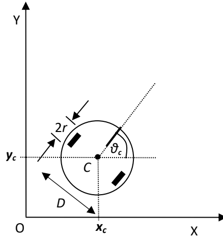
Gambar 10. Model Robot Bergerak Sederhana
